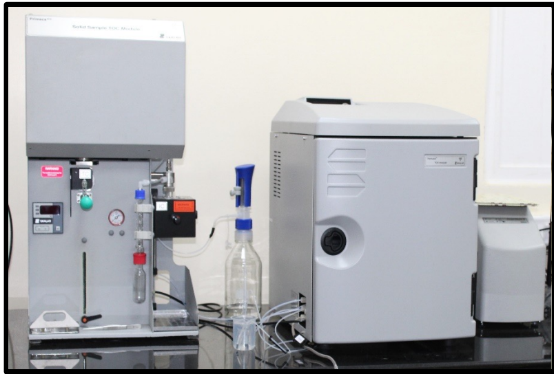
TOC Analyser
